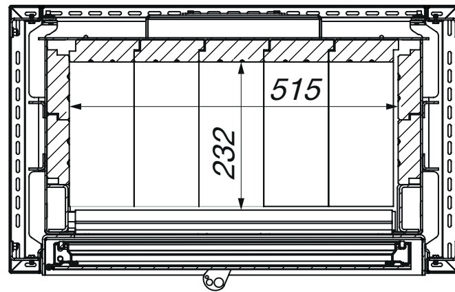
B-B (1 : 10)
