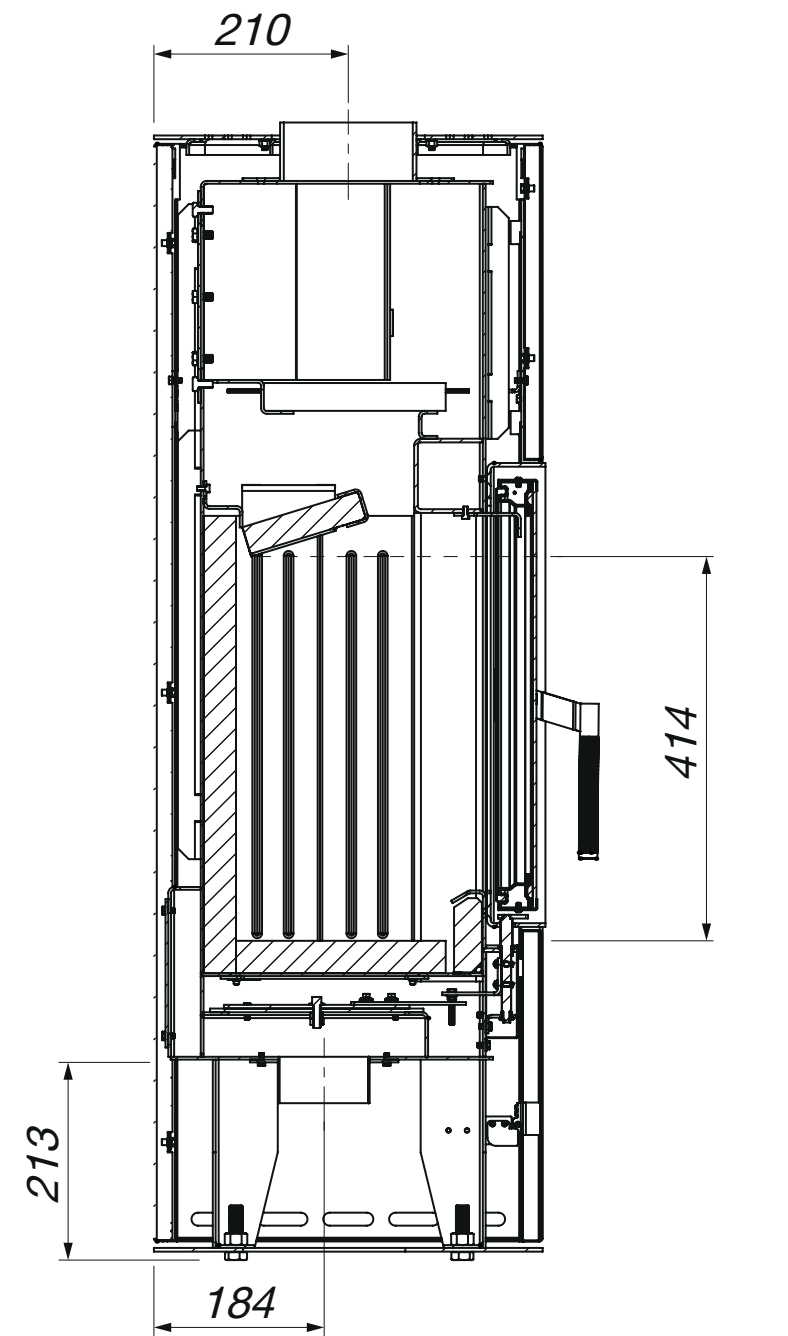
C-C (1 : 10)
