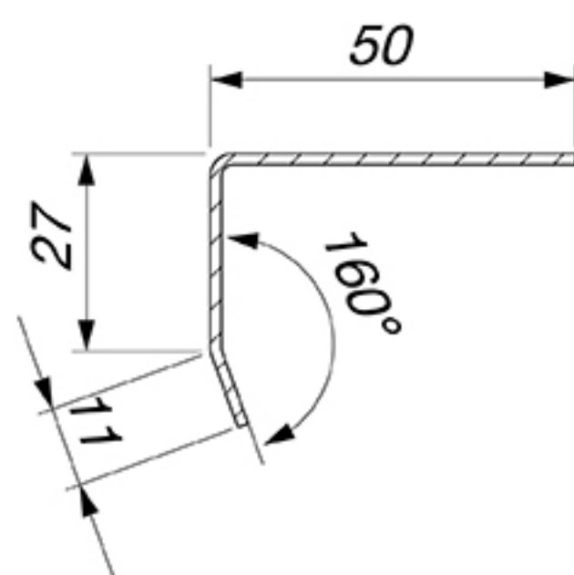
B-B (1 : 2)
