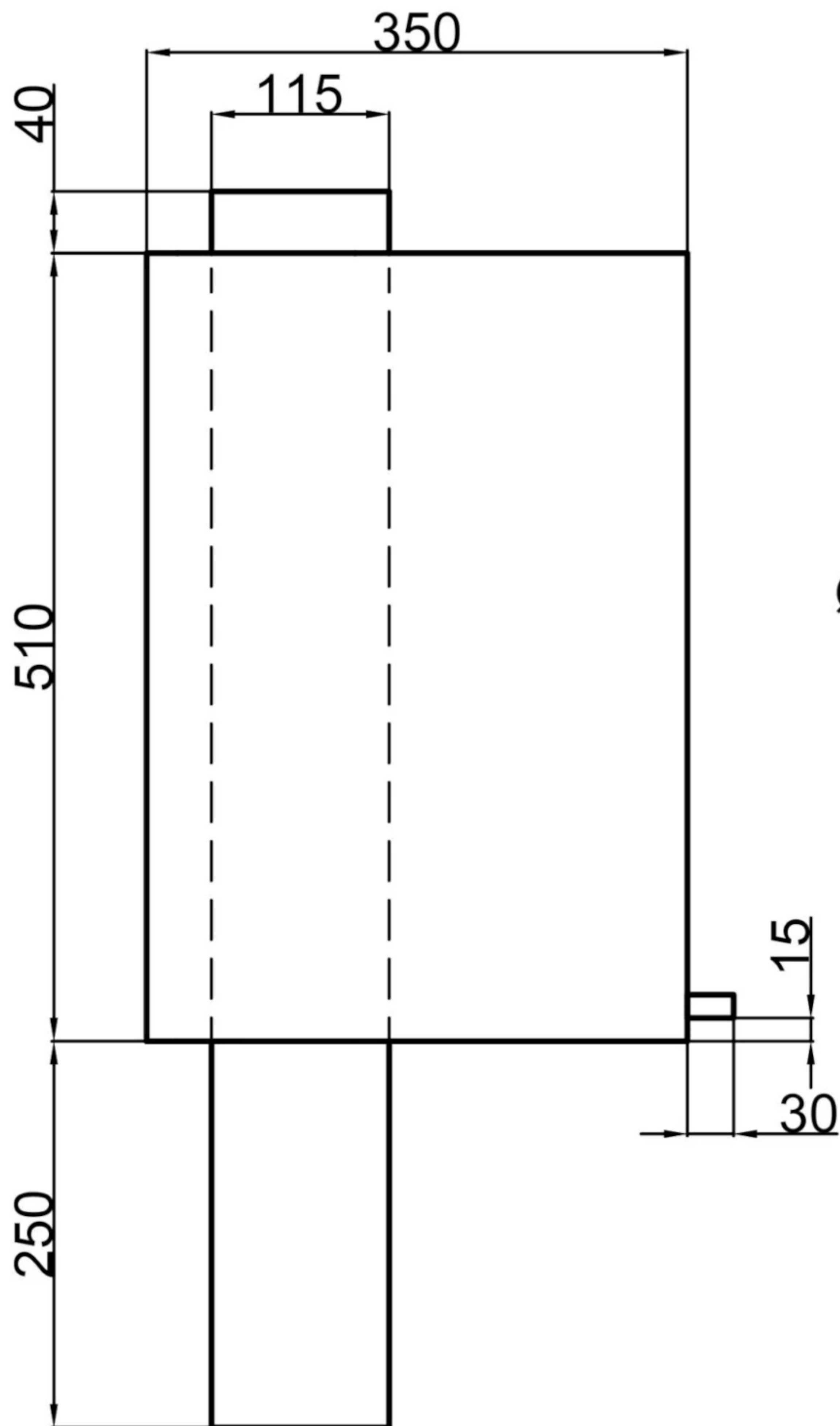
BOT-40 RV Lahtine veepaak roostevabast 40 liitrit
